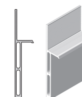
versione cartongesso
