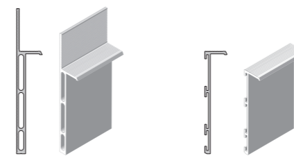
versione cartongesso (profondità 15 e 13 mm)
