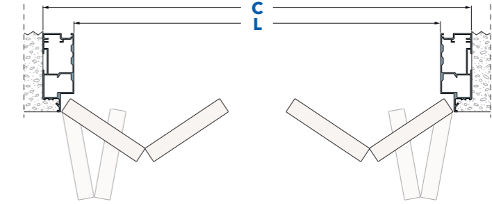
Anta a libro doppio (ogni anta è composta da due pannelli uguali)
