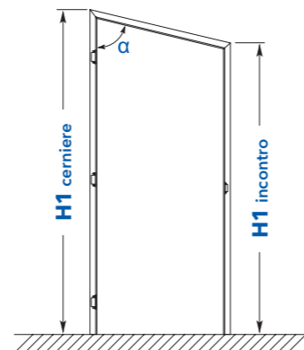
telaio battente per un'anta con o senza traverso \alpha da 60° a 89°
