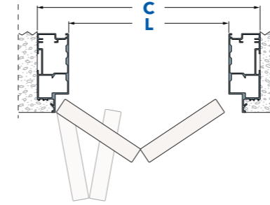
Anta a libro (l'anta è composta da due pannelli uguali)
