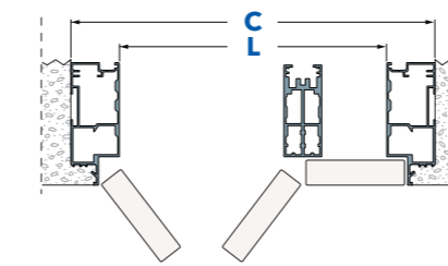
Modulare (esempio)
