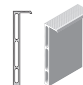
versione intonaco (profondità 15 mm)
