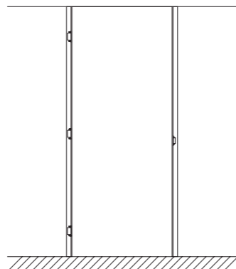
telaio battente per un'anta senza traverso (il pannello porta è a filo soffitto)
