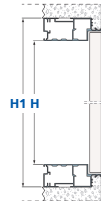
Versione a 4 lati
