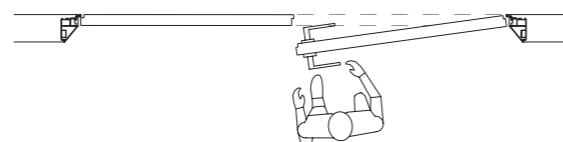
porta destra a tirare - porta sinistra fissa
